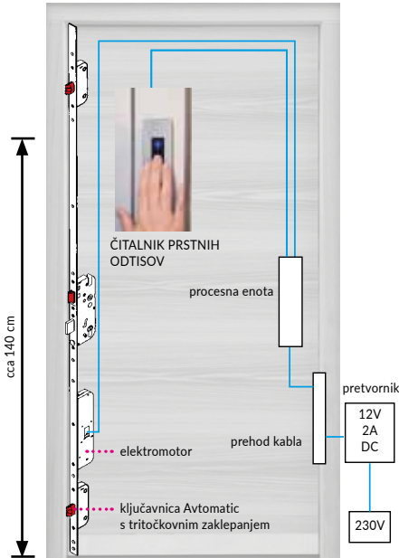
Čitalnik v držalu dLine
