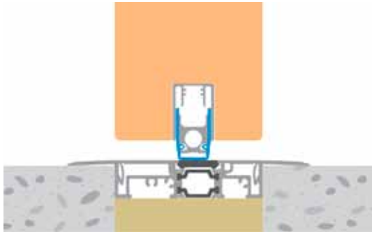
Tesnilo Planet X3, Prag Weser ZERO
