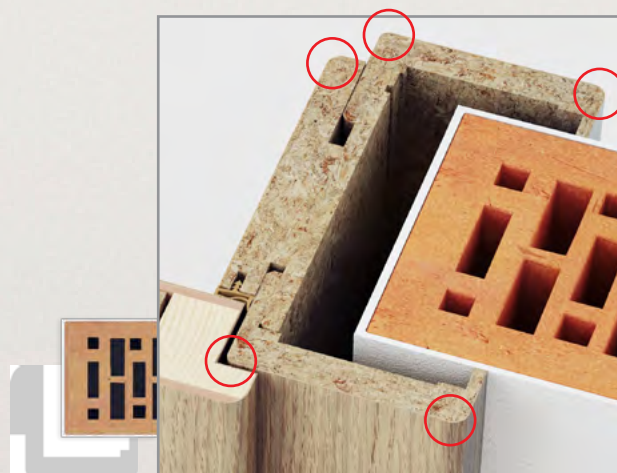
SMS podboj z vsemi zaokroženimi robovi
